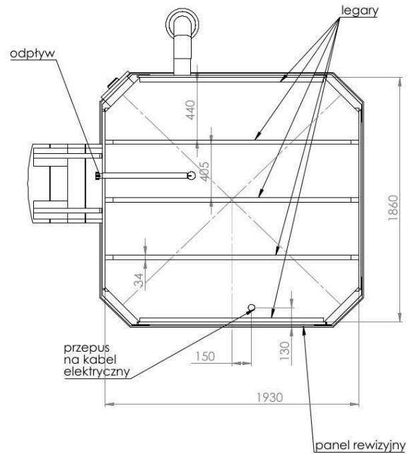
5.2 Wanna POPRAD iWE – widok od dołu
