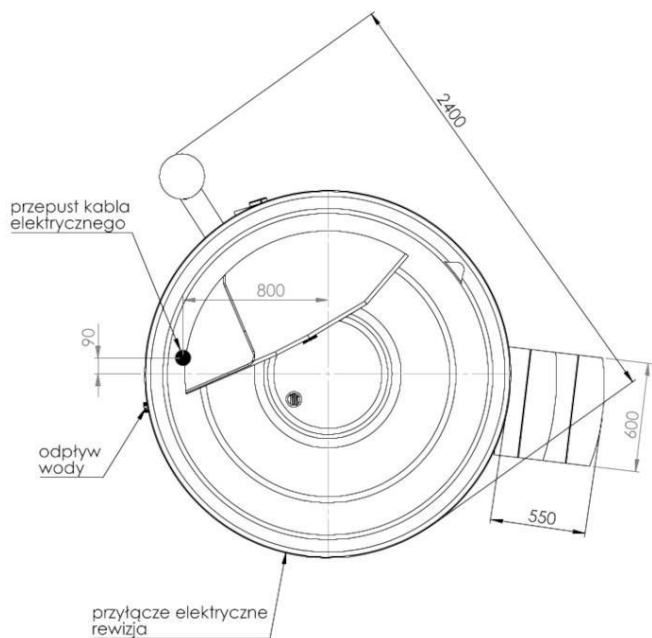
5.1 Balia OLT iWE – widok od góry
