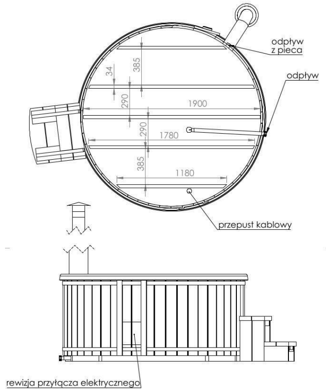
5.2 Balia OLT iW – widok od dołu
