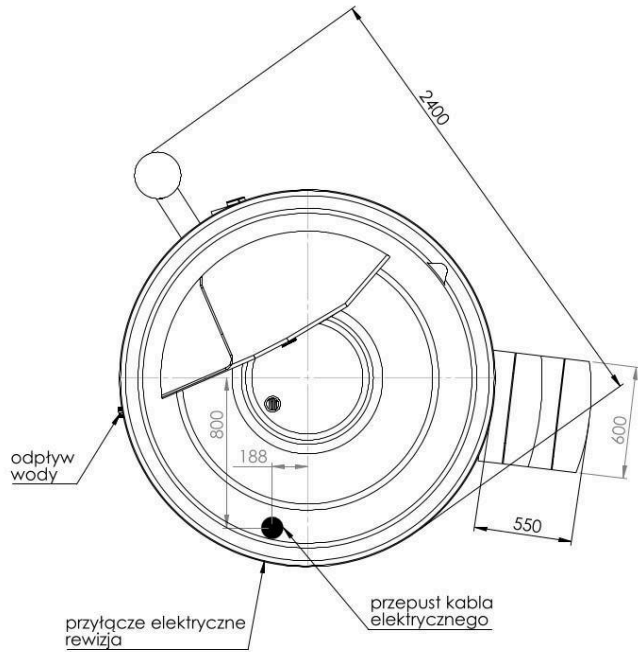
5.1 Balia OLT iW – widok od góry
