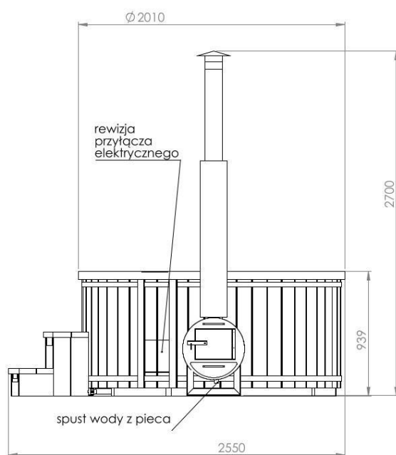
5.3 Balia CISA eW – widok od boku
